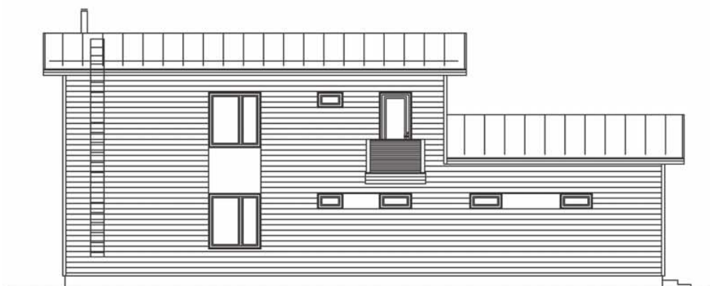
JULKISIVU POHJOISEEN
