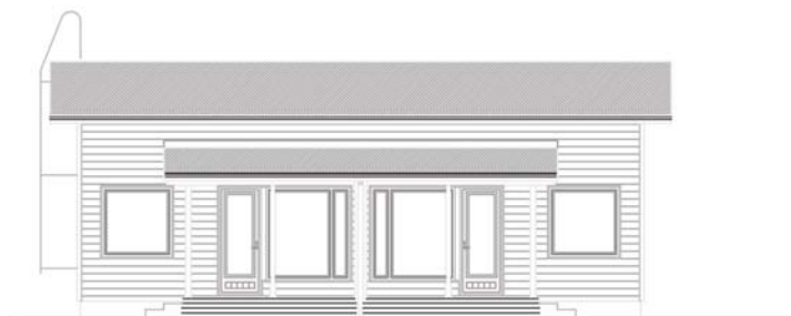
JULKISIVU KAAKKOON
