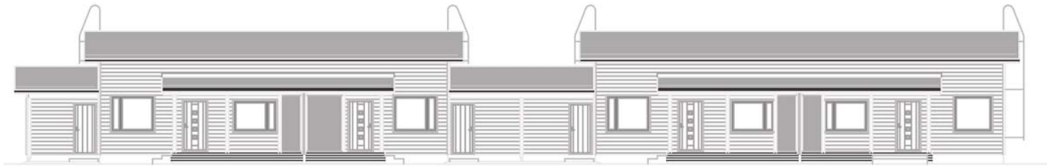
JULKISIVU KOILLISEEN
