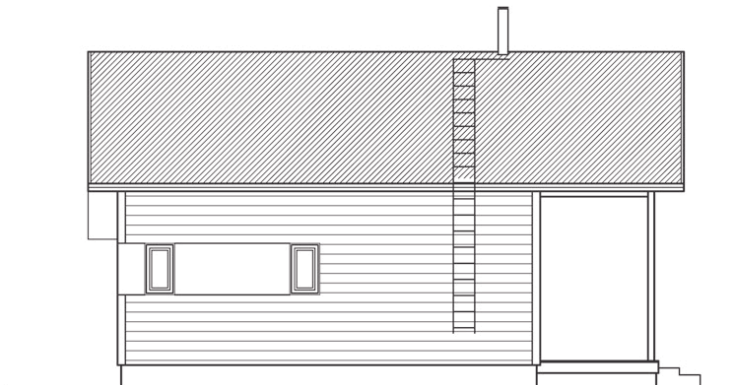
JULKISIVUT POHJOISEEN
