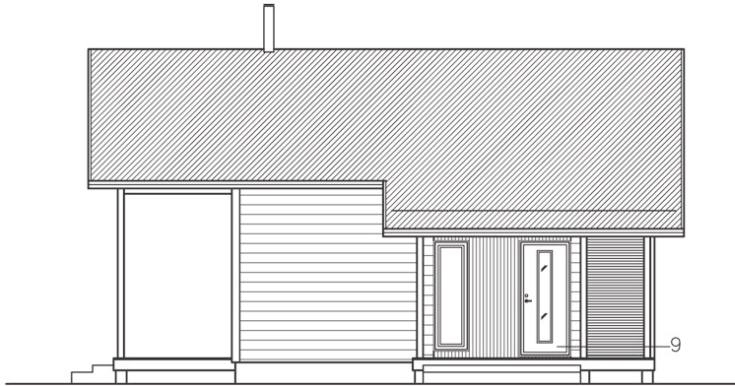
JULKISIVUT ETELÄÄN
