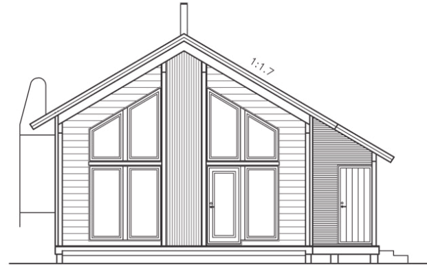
PÄÄTY LÄNTEEN
